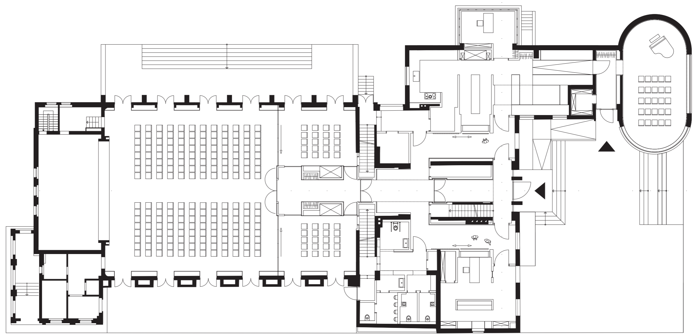
grundriss · floor plan
